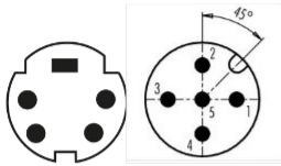
Verbindungskabel MiniDIN-Stecker-4p auf M12A-Stecker-5p (MK320) Connection cable MiniDIN-Male-4p to M12A-Male-5p
