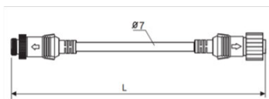
Verlängerungskabel AVS-Camera-X AI Extension cable AVS-Camera-X AI
