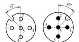
Mastkabel für Gabelstapler M12A-5p (Stecker/Busche) Mast cable for Forklift M12A-5p (Male/Female)
